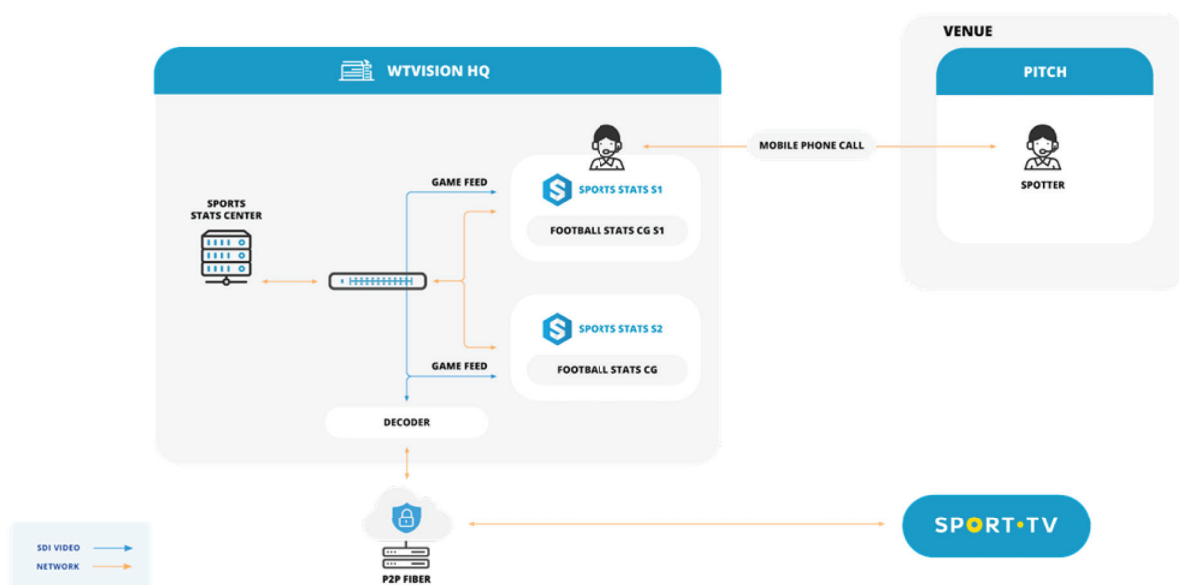
Figura 12: Diagrama simplificado del proceso de recolección remota de datos para los juegos de la Liga Portugal.
