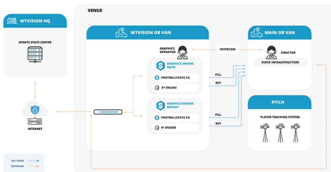
Figura 2: Diagrama de operaciones y servicios - locales y remotos - durante un partido de la Liga Portugal.
